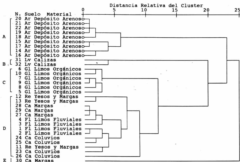
Figura 1.- Dendograma entre grupos.
