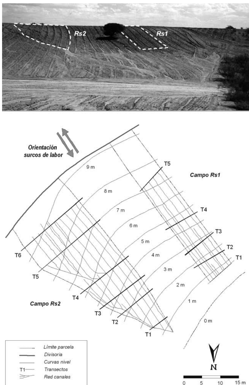
FIGURA 4: Formaciones de regueros en una ladera agrícola en condiciones de Barbecho convencional (Barbecho blanco). La orientación de los surcos de labor es paralela a la dirección de la máxima pendiente en el campo Rs1 y según una dirección oblicua a la de máxima pendiente en el campo Rs2 (Rielves, Toledo).
