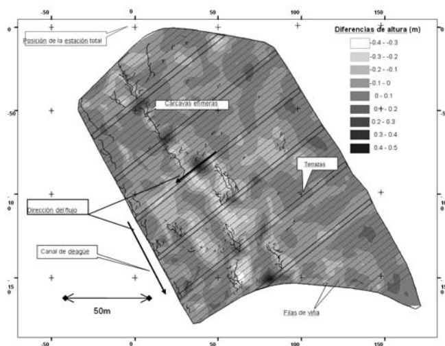
FIGURA 2: Mapa de redistribución y pérdidas de suelo obtenido por sustracción de modelos digitales de dos fechas.
