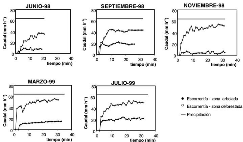
FIGURA 1: Hidrogramas de las experiencias con lluvia simulada.
