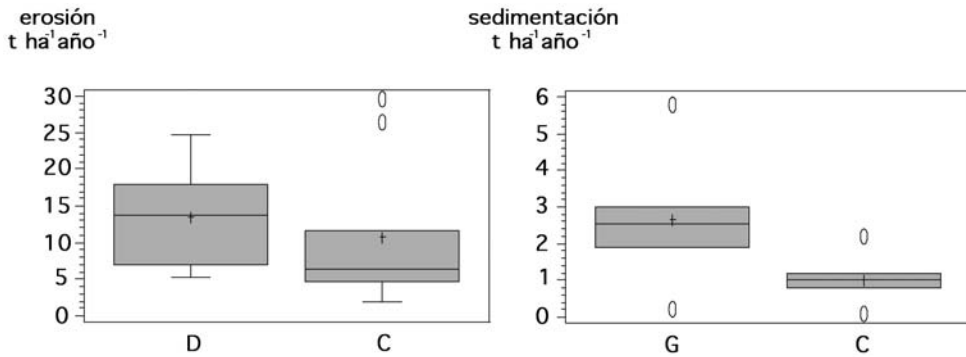
FIGURA 1: Gráficos box-whisker de las velocidades de erosión y sedimentación calculadas con los distintos modelos aplicados.
