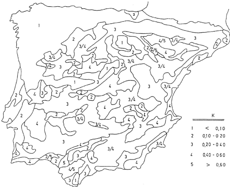
Figura 1. Clases de erosionabilidad de las unidades FAO (1985) de los suelos españoles (factor K de la USLE).
