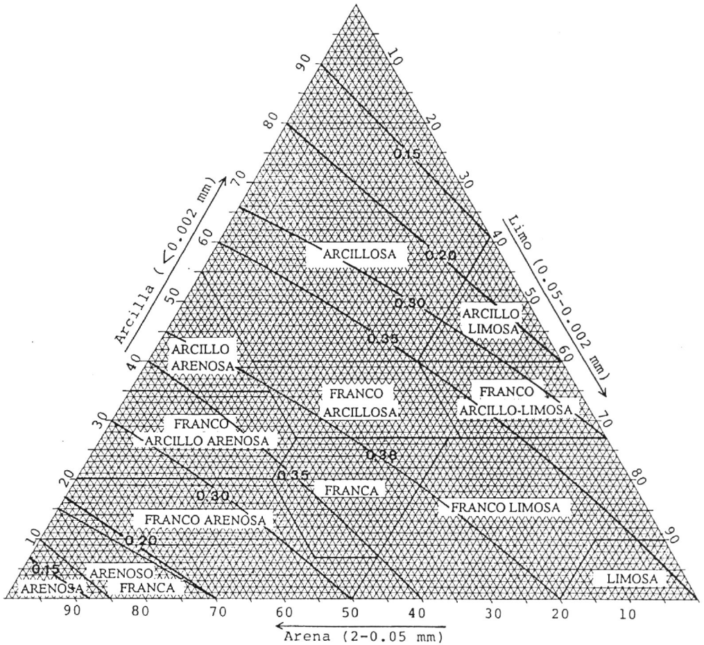
Figura 2. Relación entre el factor K según la versión simplificada de la RUSLE y las clases de textura USDA.
