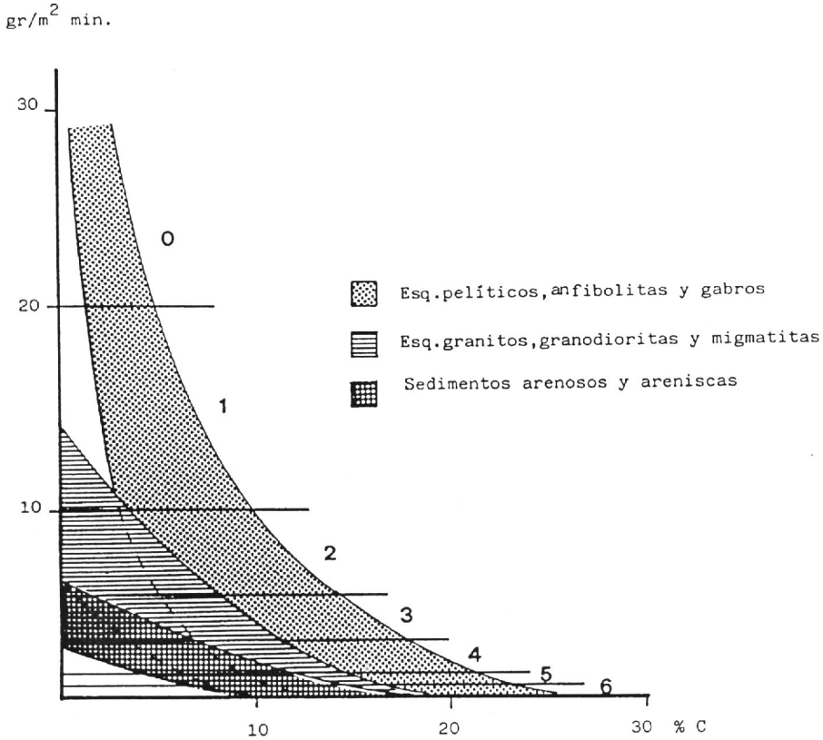
Figura 3. Relación entre la erosionabilidad de suelos de la zona húmeda española y su contenido en materia orgánica (Díaz-Fierros y Benito, 1991).
